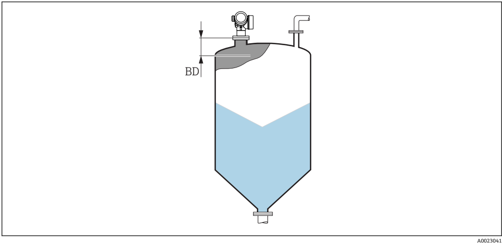
40 料位测量时的盲区距离 (BD)
