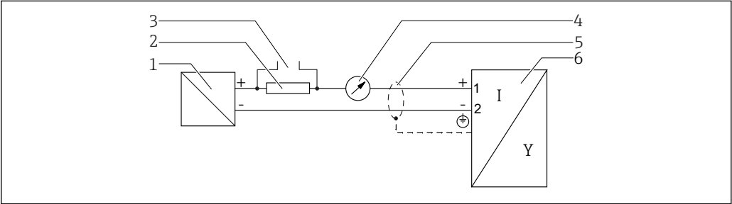
8 接线图: 两线制; 4...20 mA HART
