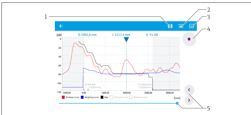
图 29 在 SmartBlue 中显示包络线；Android 视图
