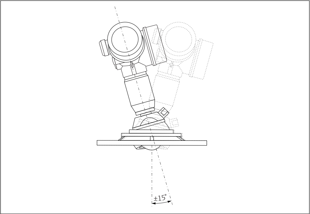
6 带天线角度调节装置的 Micropilot FMR67
