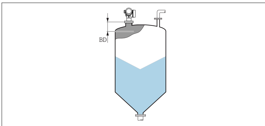
图 44 固体测量时的盲区距离 (BD)
