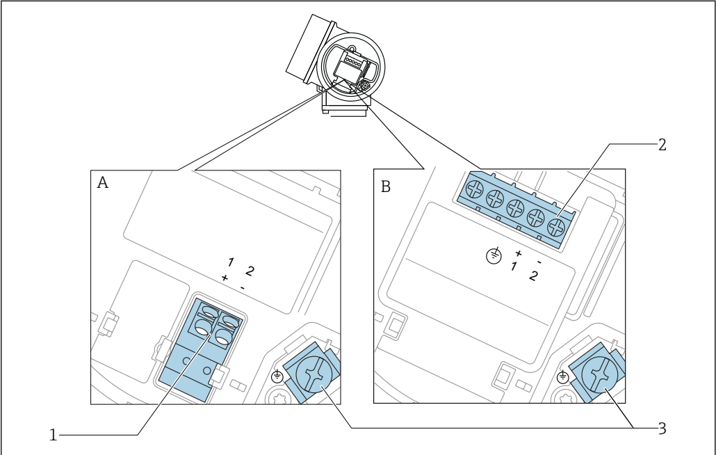
7 接线端子分配: 两线制; 4...20 mA HART
