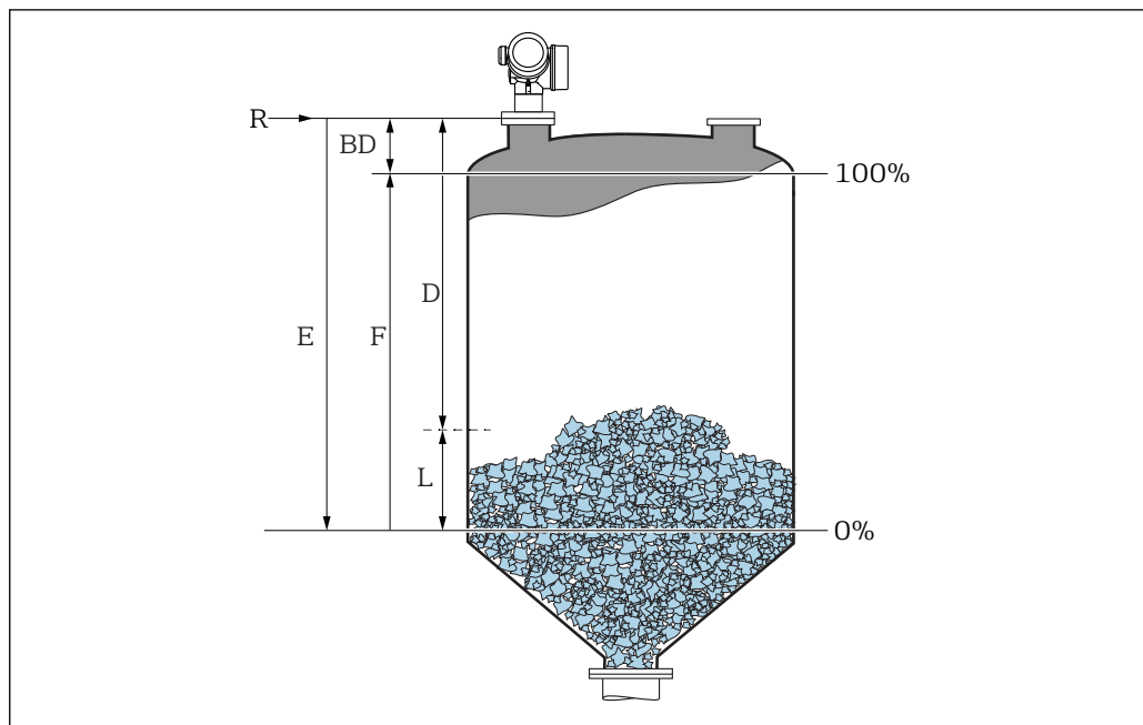
图 32 料位测量时的设置参数
