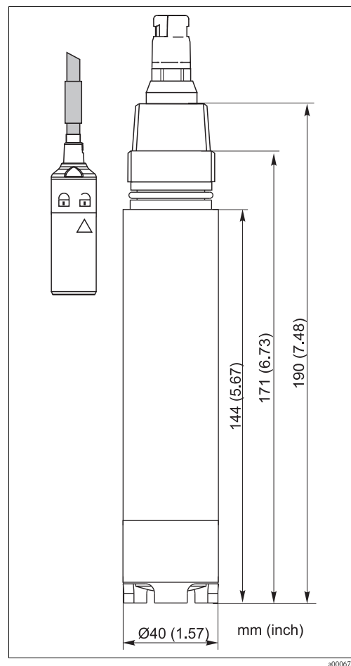
Fig. 1: Dimensions
