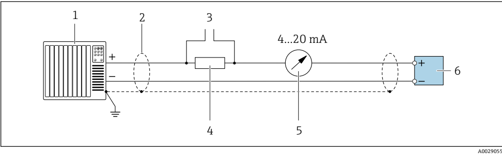
图 39 接线示例：4...20 mA HART 电流输出（有源信号）
