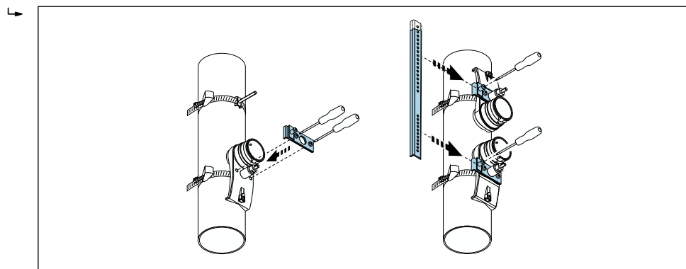
31 安装传感器安装支座和安装轨
