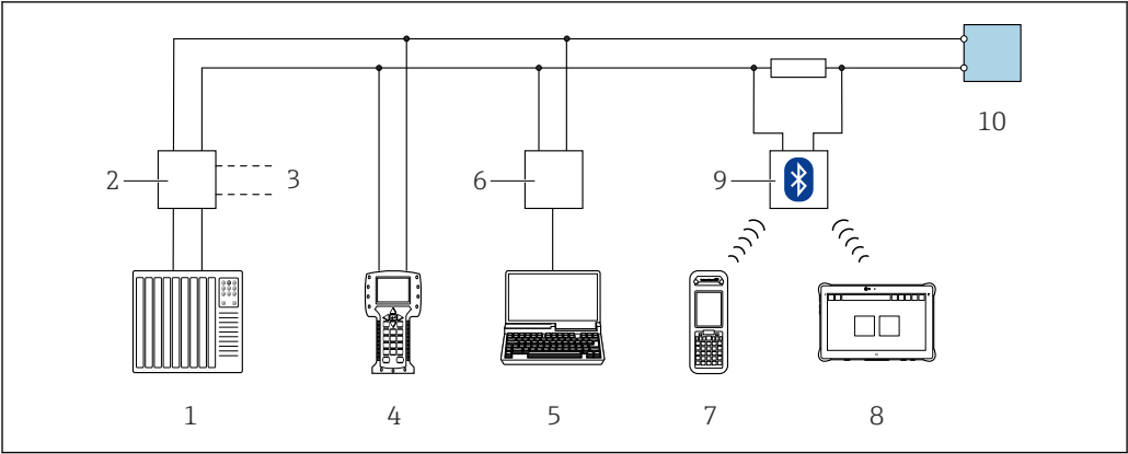
56 通过 HART 通信进行远程操作（无源信号）
