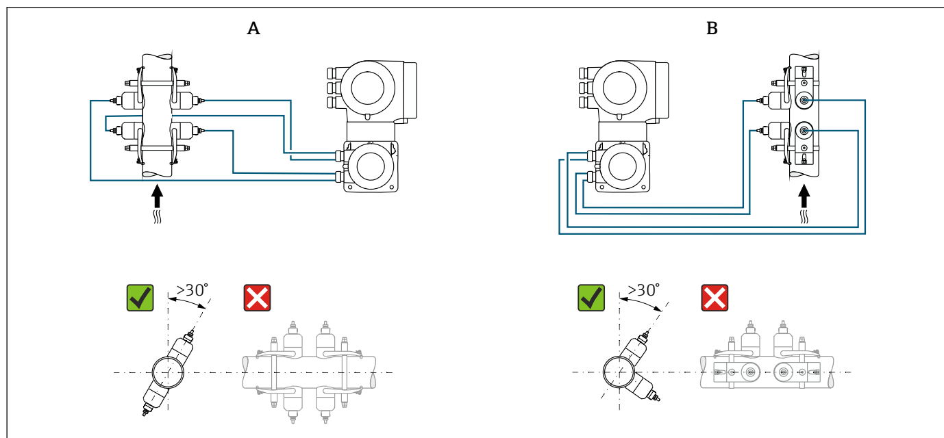
图 7 双声路测量：传感器套件在测量点处水平布置实例
