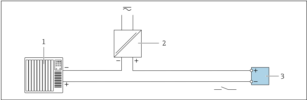
图 48 继电器输出的连接实例(无源) 1 带继电器输入的自动化系统(例如： PLC) 2 电源 3 变送器：注意输入参数→ 167
