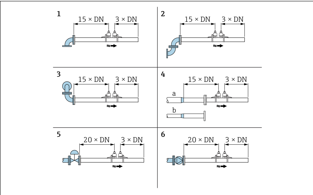
图 6 使用不同节流装置时的最小前后直管道长度
