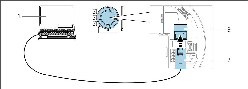
57 通过服务接口（CDI-RJ45）连接
