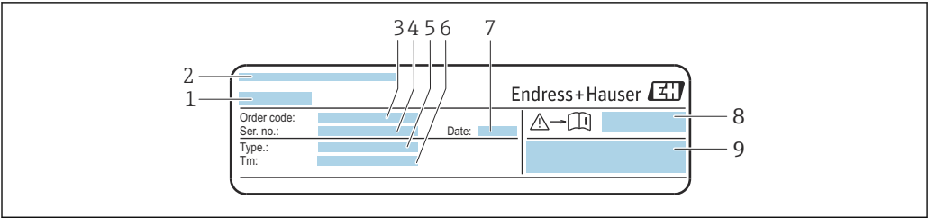
3 传感器的铭牌示意图，“正面” 1 传感器型号 2 制造地 3 订货号 4 序列号 5 类型 6 介质温度范围 7 生产日期：年-月 8 《安全指南》补充文档资料代号→ 182 9 附加信息
