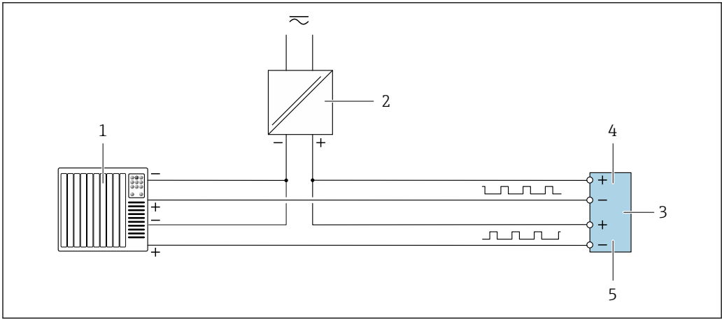
图 47 脉冲（相移）输出的连接实例（无源信号） 1 带脉冲（相移）输出的自动化系统（例如 PLC） 2 电源 3 变送器：注意输入参数 4 脉冲输出 5 脉冲（相移）输出（从设备）
