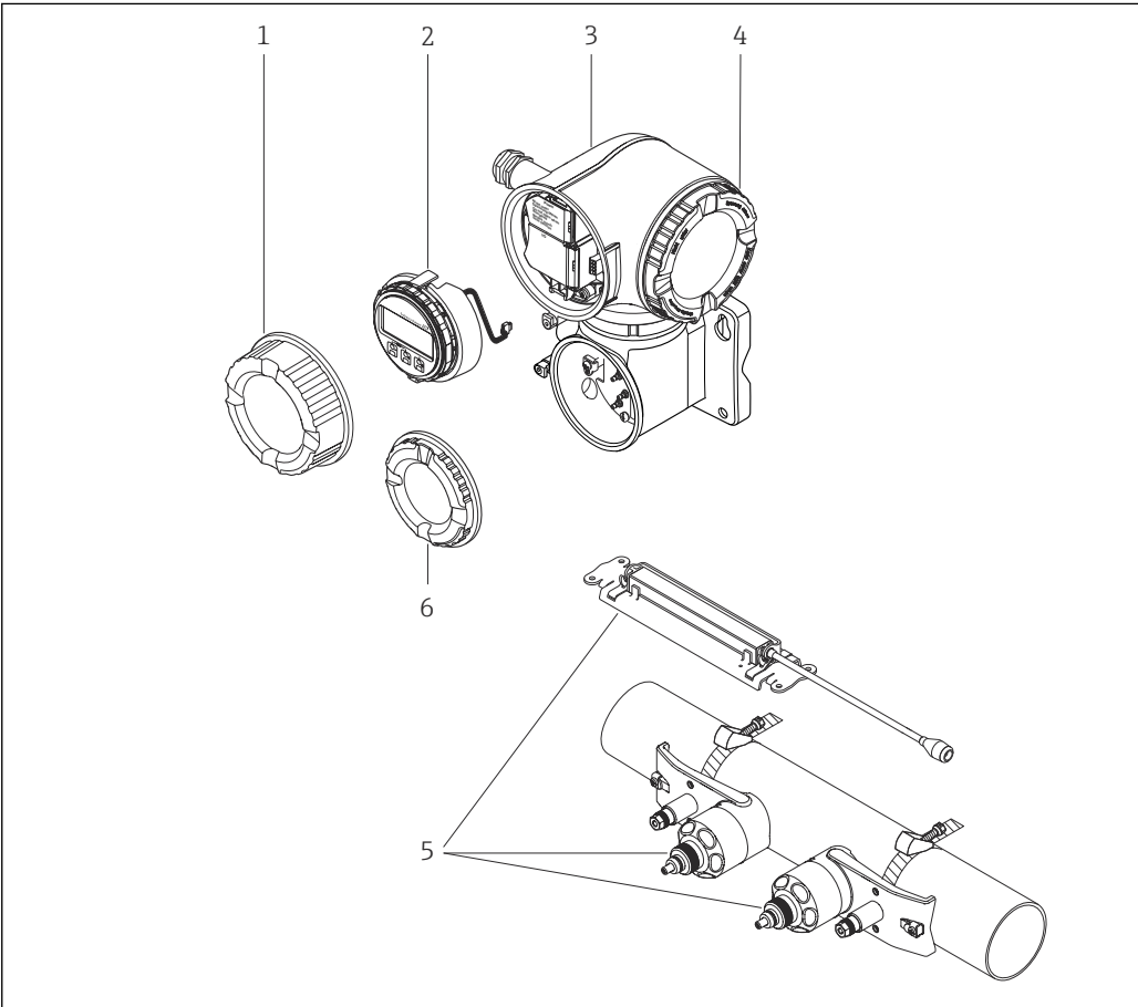
1 仪表的主要组成部件
