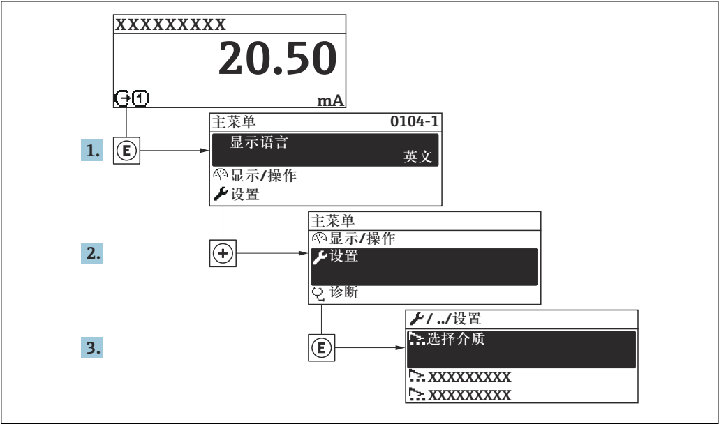
59 现场显示单元示例
