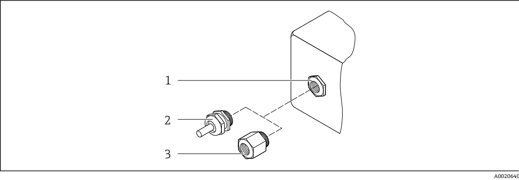
图 68 允许的电缆入口/缆塞
