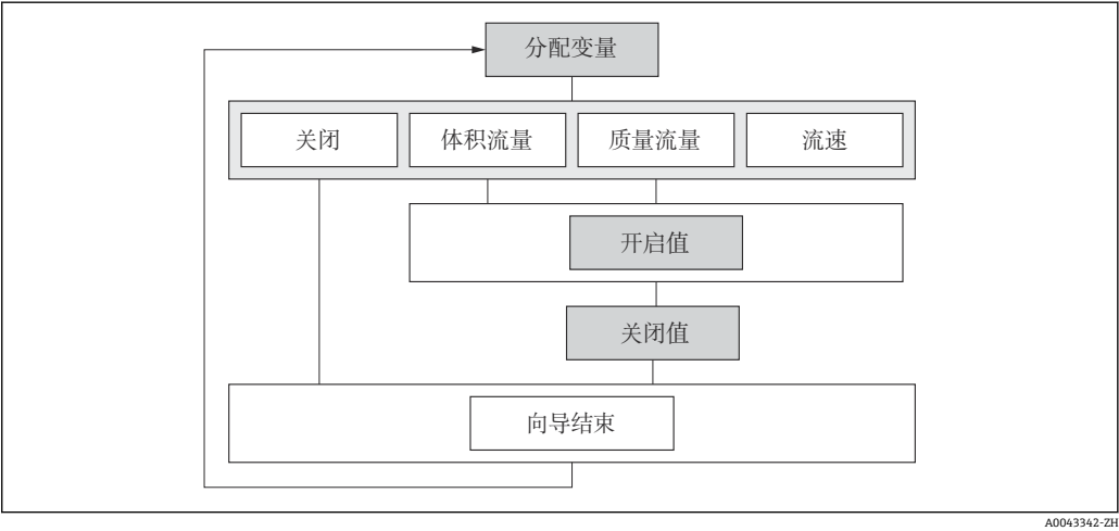
图 61 “设置”菜单中的“小流量切除”设置向导
