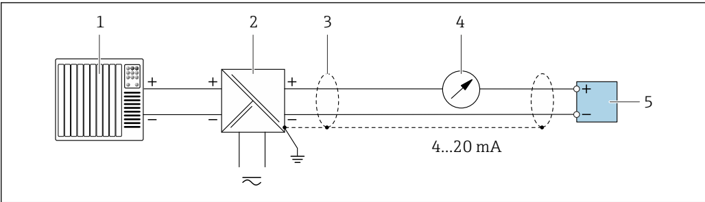
图 40 接线示例：4...20 mA HART 电流输出（无源信号）
