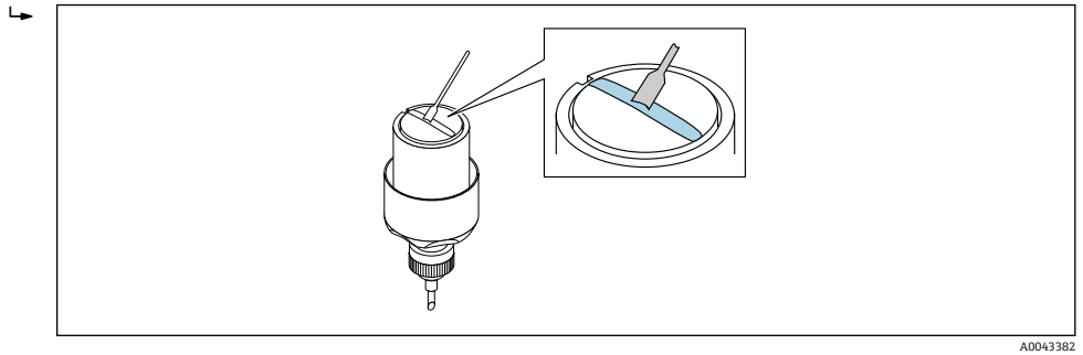
图 28 在传感器的接触面上涂抹耦合凝胶（如果没有耦合垫）
