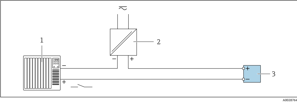
图 50 状态输入的连接示例 1 带状态输出的自动化系统（例如 PLC） 2 电源 3 变压器
