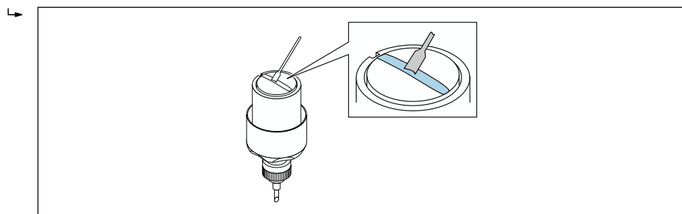
32 在传感器的接触面上涂抹耦合凝胶 (如果没有耦合垫)
