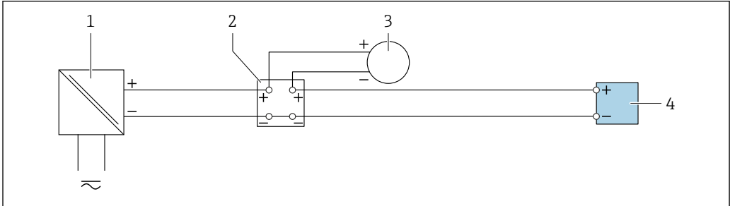
图 49 4...20 mA 电流输入的连接示例 1 电源 2 接线盒 3 外接测量设备（例如用于读取压力或温度值） 4 变送器
