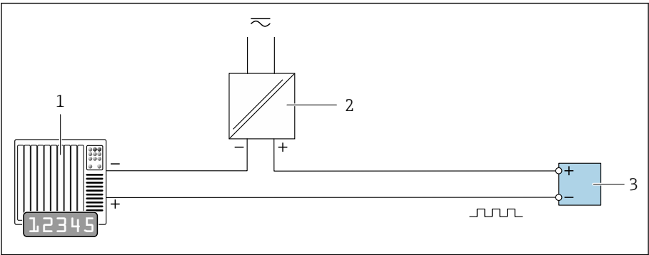
1 自动化系统，带脉冲输出和频率输入（例如 PLC） 2 电源 3 变送器：注意输入参数。
