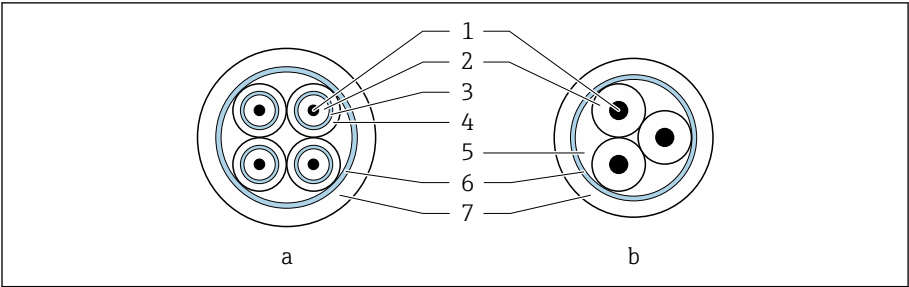
8 电缆截面图
