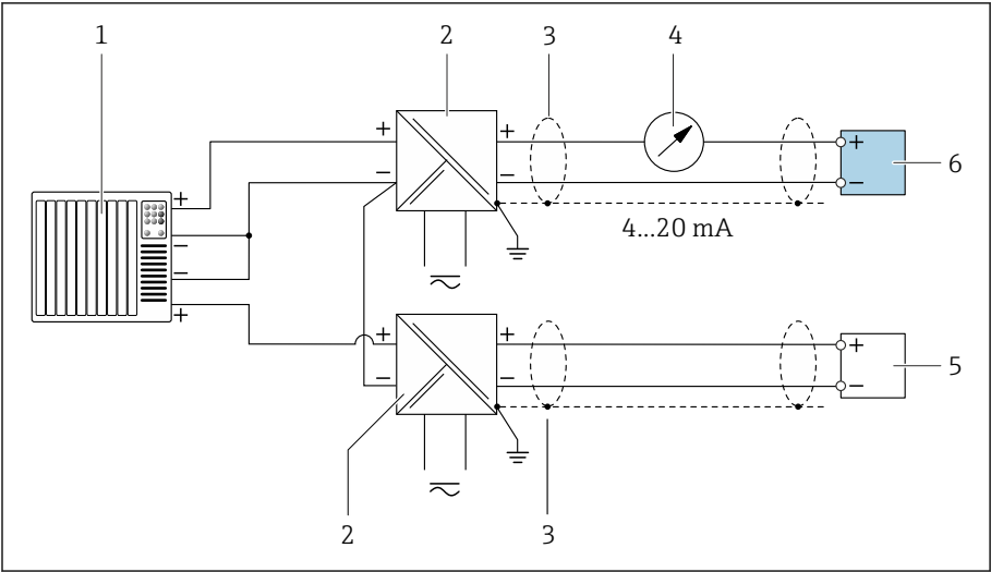
10 接线示例，HART 输入，公共端接负极（无源信号） 1 自动化系统，带电流输入（例如 PLC） 2 电源安全栅（例如 RN221N） 3 电缆屏蔽层 4 模拟式显示单元：注意最大负载。 5 压力测量仪表（例如 Cerabar M、Cerabar S）；注意相关要求 6 变送器
