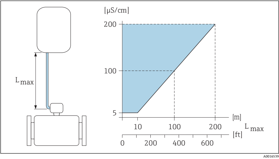
9 允许连接电缆长度 彩色区域 = 允许电缆长度范围 L_{max} = 连接电缆长度 ([m] ([ft]) ) [µS/cm] = 介质电导率
