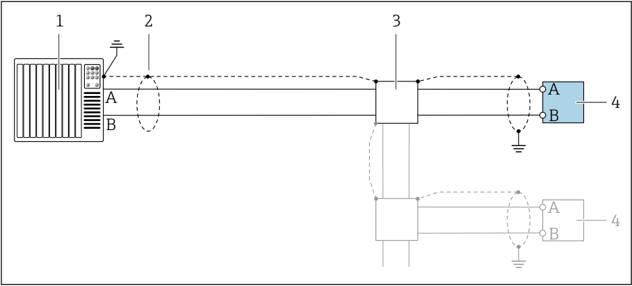
11 接线示例，Modbus RS485，非防爆区和防爆区（Zone 2；Cl. I, Div. 2）
