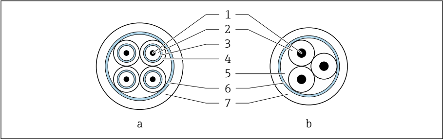
图 9 电缆截面图
