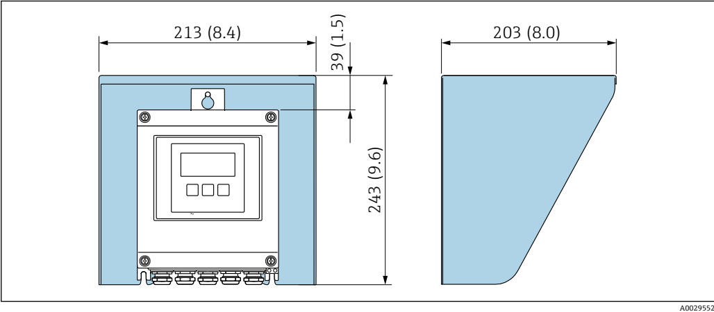
图 9 Proline 500 (数字) 的防护罩
