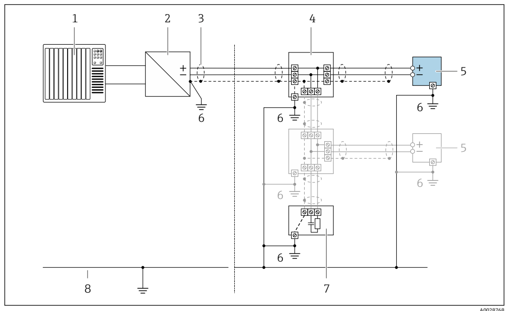
图 23 基金会现场总线 (FF) 的连接实例
