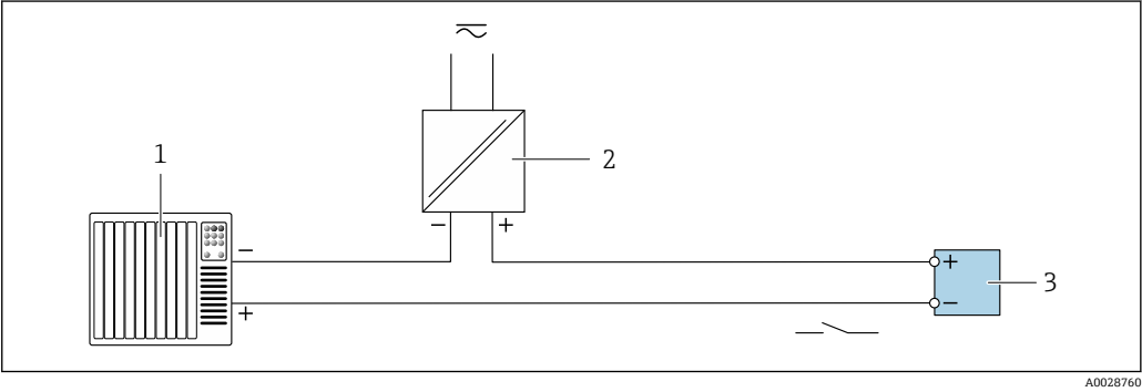
图 28 继电器输出的连接实例(无源)
