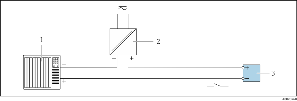
图 27 开关量输出(无源信号)的连接实例
