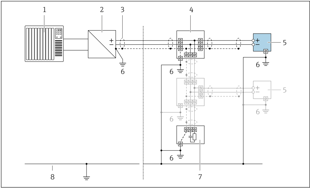
图 17 FOUNDATION Fieldbus 的接线实例
