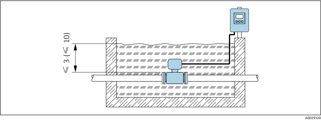
图 11 单位: m (ft)
