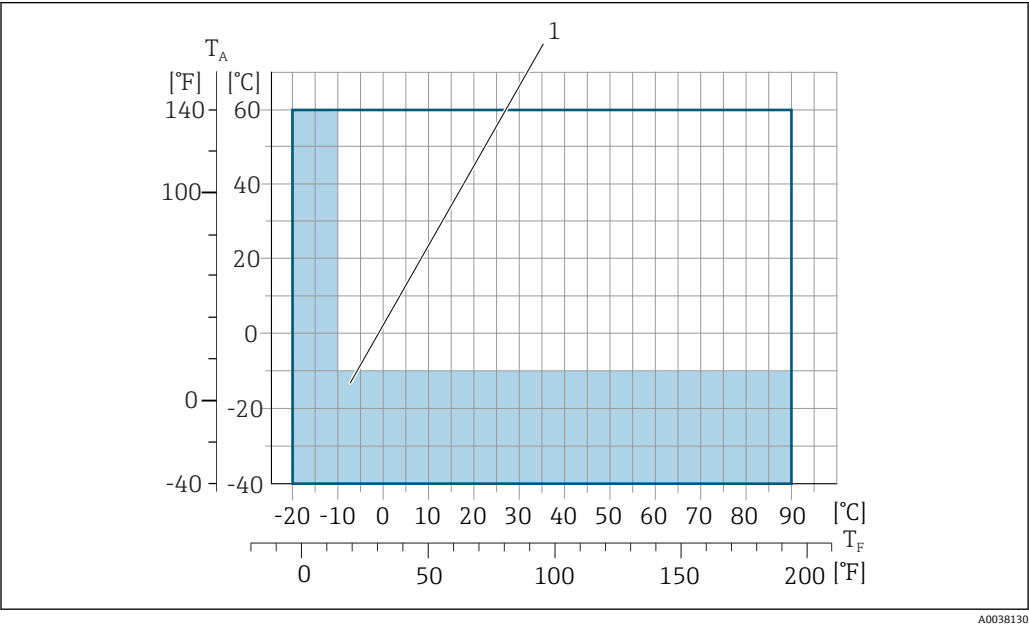
T A 环境温度范围 T F 流体温度 1 彩色区域：环境温度范围-10 ... -40 °C (+14 ... -40 °F)；流体温度范围-10 ... -20 °C (+14 ... -4 °F)（仅适用不锈钢法兰）
