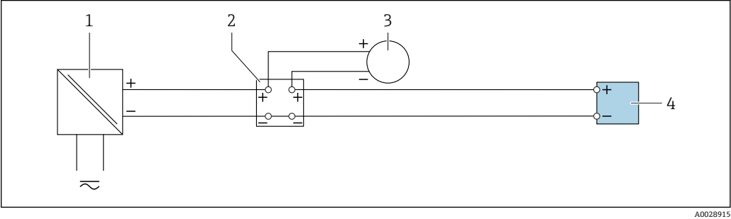
图 29 4...20 mA 电流输入的连接示例
