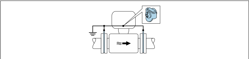
22 通过接地端子和接地环实现系统电势平衡
