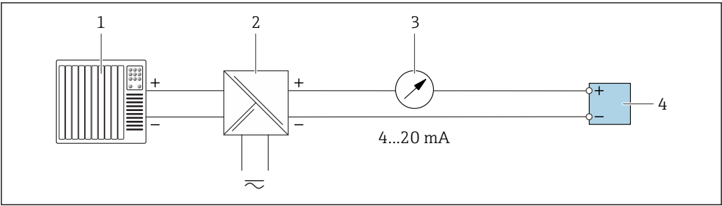
图 25 4...20 mA 电流输出（无源）的连接示例
